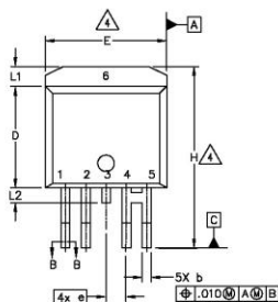
VIEW A-A
