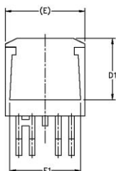
VIEW A-A
