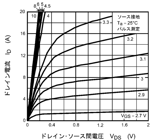
図 8.2 I_D - V_{DS}
